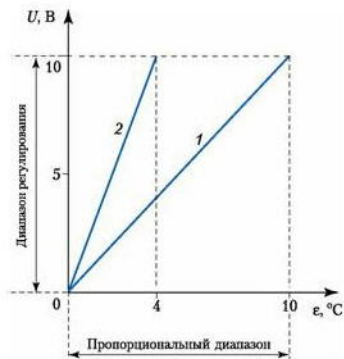
Рис. 2.12. График пропорционального регулирования
