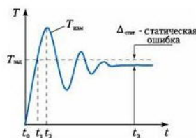
Рис. 2.13. Переходной процесс при пропорциональном (П) регулировании
