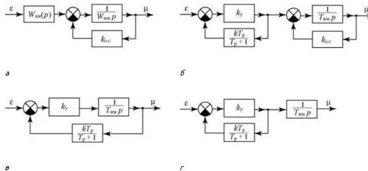
Рис. 2.20. Структурные схемы промышленных ПИ-регуляторов
