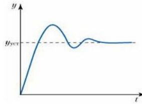
Рис. 2.22 Переходной процесс при ПИД-регулировании
