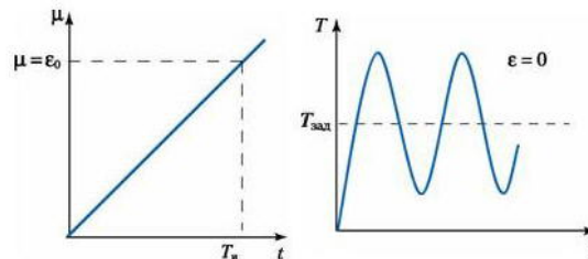
Рис. 2.16. Закон регулирования (а) и переходной процесс (б) при интегральном (И) регулировании
