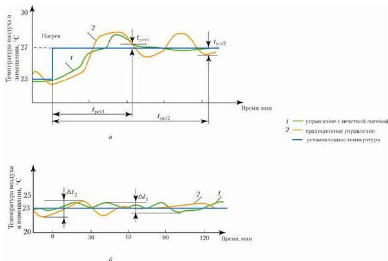
Рис. 2.27. Графики изменения температуры в помещении а — кривая разгона; б — изменение температуры в помещении
