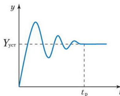
Рис. 2.19. Переходной процесс при пропорционально-интегральном (ПИ) регулировании
