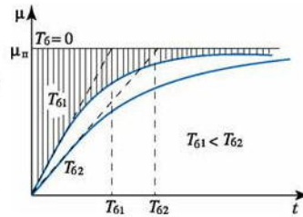
Рис. 2.15. Закон П-регулирования
