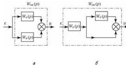
Рис. 2.17. Структурная схема идеальных ПИ-регуляторов: а – с передаточной функцией (2.12); б – с передаточной функцией (2.14)
