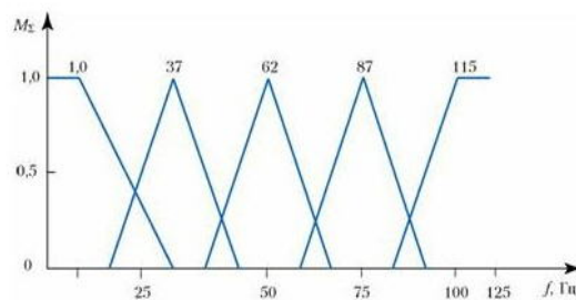
Рис. 2.25. Зависимость параметра "частота вращения компрессора" от значения суммарной функции принадлежности
