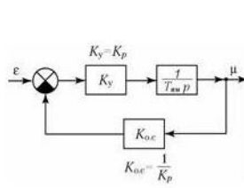
Рис. 2.14. Структурная схема П-регулятора
