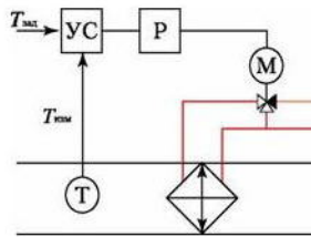
Рис. 2.11. Контур регулирования температуры приточного воздуха в канале центрального кондиционера
