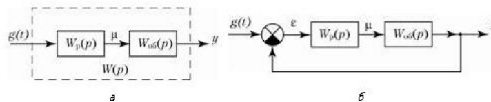
Рис. 2.10. Структурная схема САР: а – разомкнутой системы по каналу задающего воздействия; б – то же, но замкнутой системы
