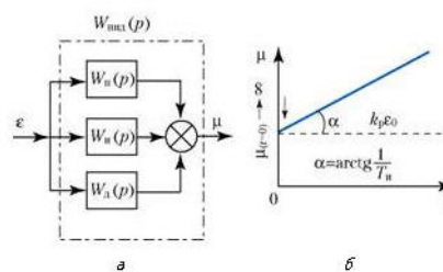
Рис. 2.21. Структурная схема ПИД-регулятора (а) и закон ПИД-регулирования (б)
