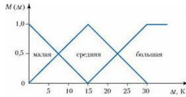
Рис. 2.23. Функция принадлежности для лингвистического аргумента "разность температур"
