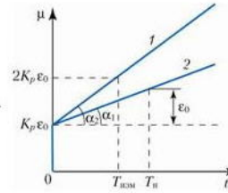
Рис. 2.18. Закон ПИ-регулирования регуляторов 1 – с передаточной функцией (2.12) 2 – с передаточной функцией (2.14)
