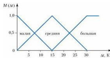
Рис. 2.4. Функция принадлежности для лингвистического аргумента "скорость изменения температуры"
